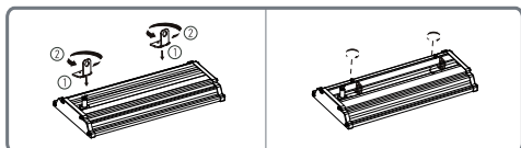
2. Установка настенной части кронштейна на монтажной поверхности
