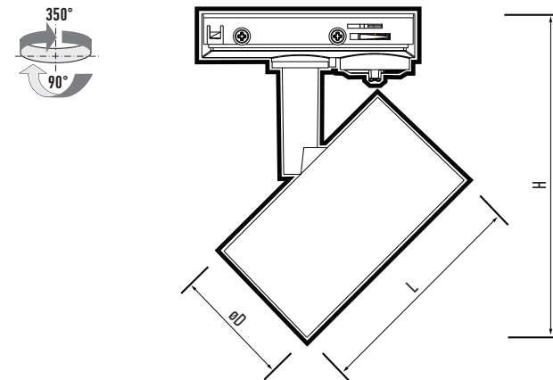
Рис. №1 Светильник PTR 36
